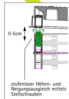
höhenverstellbar
