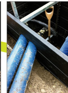
schräge Rohranbindung
