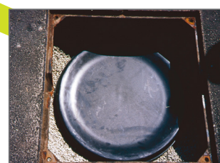
Dichtes Schachtabdeckungssystem mit getrennter Dicht- und Tragfunktion
