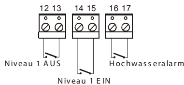
Betrieb mit 3 Schwimmschaltern
