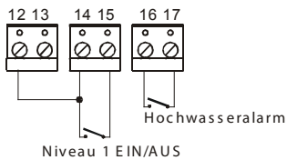
Betrieb mit 2 Schwimmschaltern
